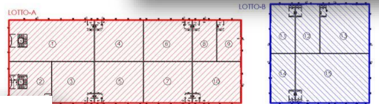
nel progetto preliminare architettonico, dei due volumi componenti l'insediamento industriale (piano terra).
